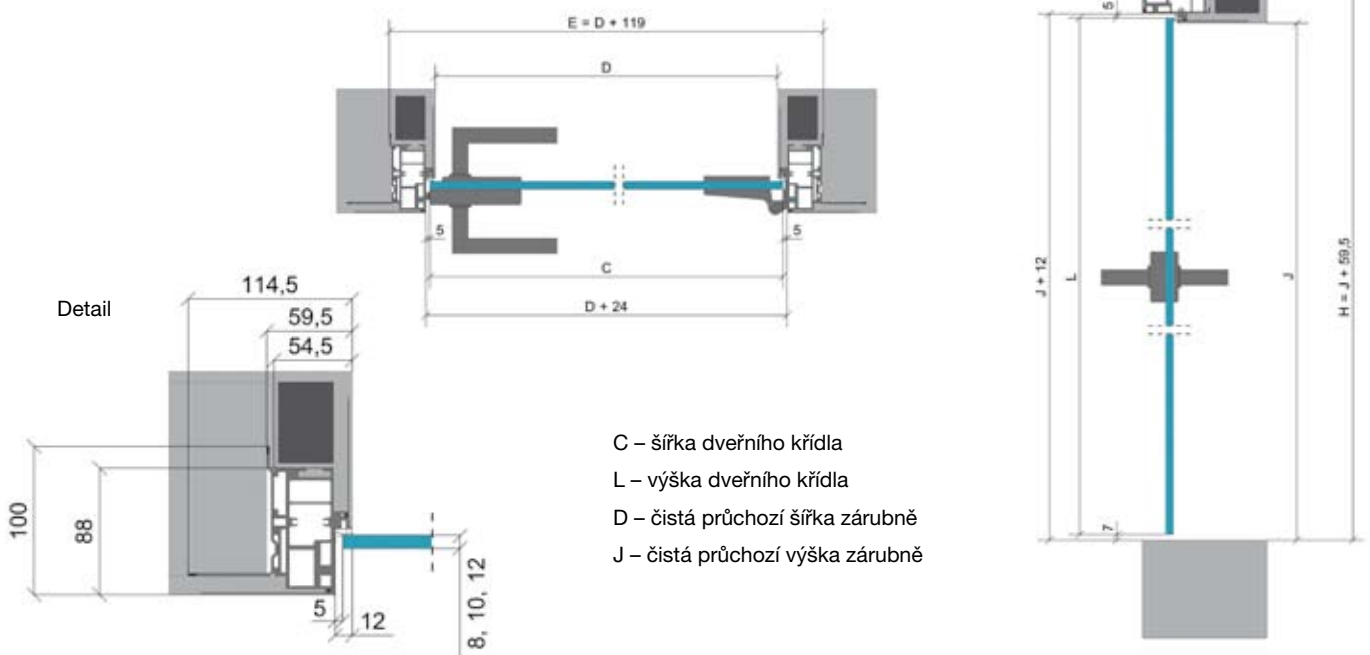
SKLENĚNÉ DVEŘE
