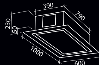
Recirkulačná verzia
