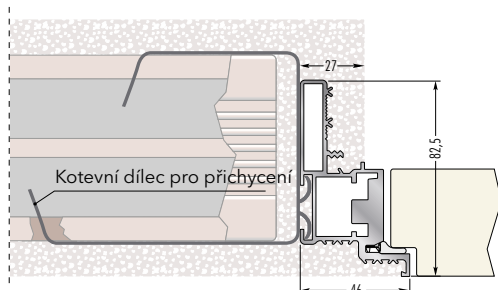
Zárubeň do zdiva
