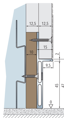
Soklový profil na SDK stěně při dvojitým opláštění.
