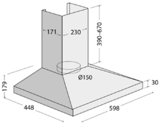
OPV3660
