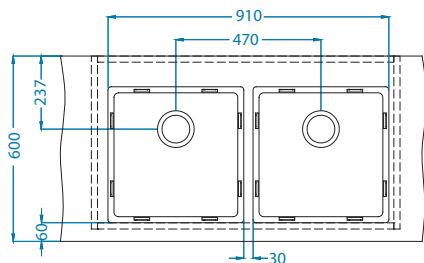
KOMBINO 30 - 2X
