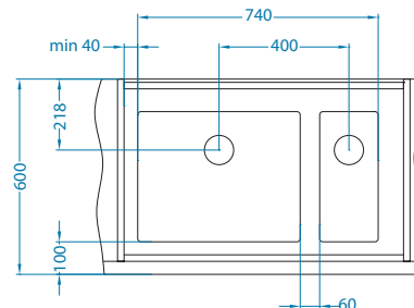
QUADRIX 10+50-U
