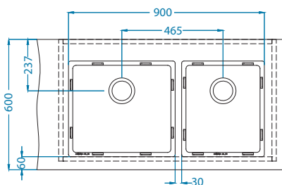
KOMBINO 40 + KOMBINO 20
