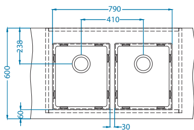
KOMBINO 20 - 2X
