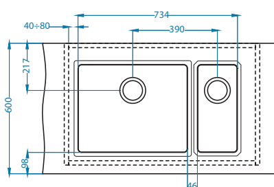
KOMBINO 50 + KOMBINO 10
