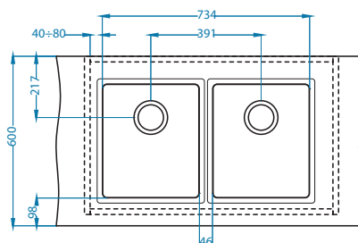
KOMBINO 20 - 2X
